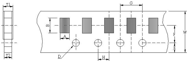
0402&0603 4P2R 8P4R 10P8R D Type
